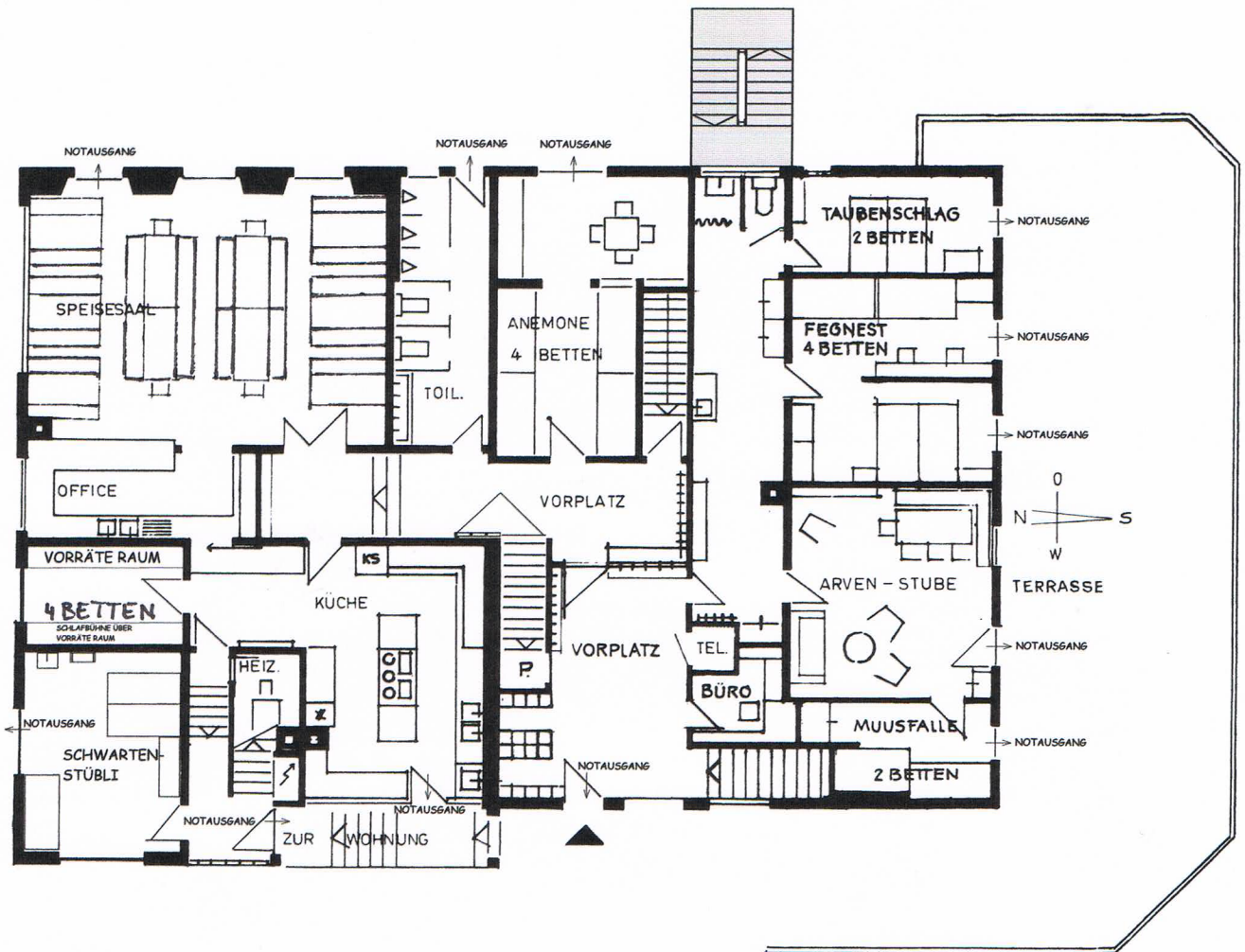
Grundriss Erdgeschoss
